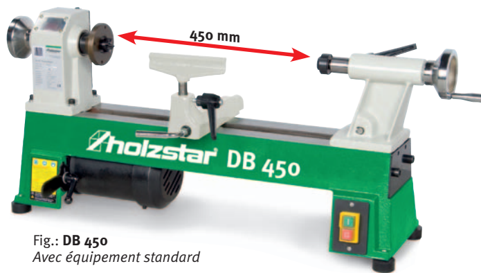
Fig.: DB 450 Avec extension de banc en option portant l'entrepointe à 1000 mm Code article 592 0451
